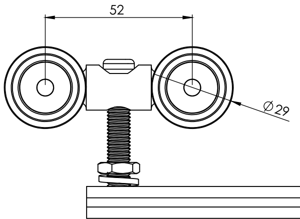
ROLD R4-150 CE Roldana simples CE 150Kg
