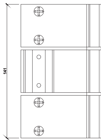
DOB-BR01T Dobradiça de Balanço Tripla Máximo 90kg por folha 4 unidades
