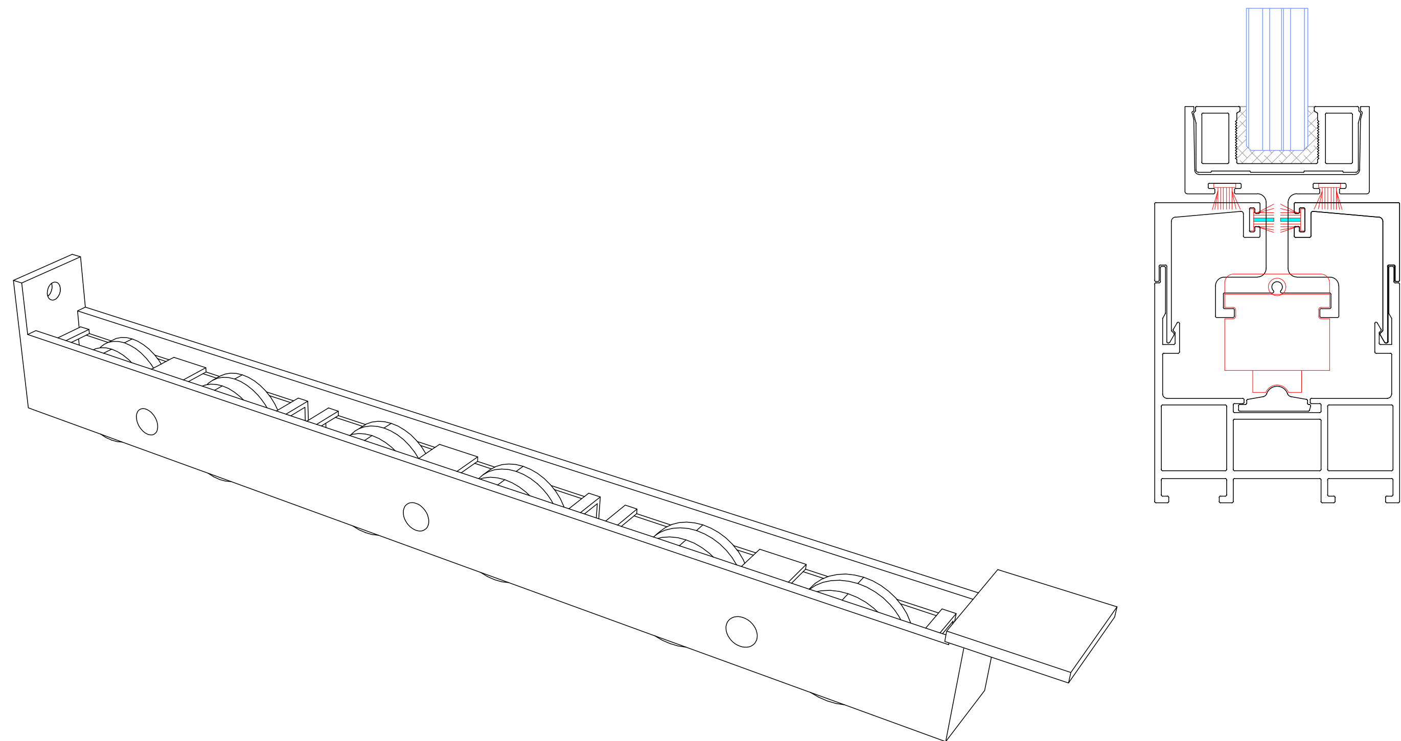
ROLD-MD.6R Roldana Minimal 3 com 6 Rodas
