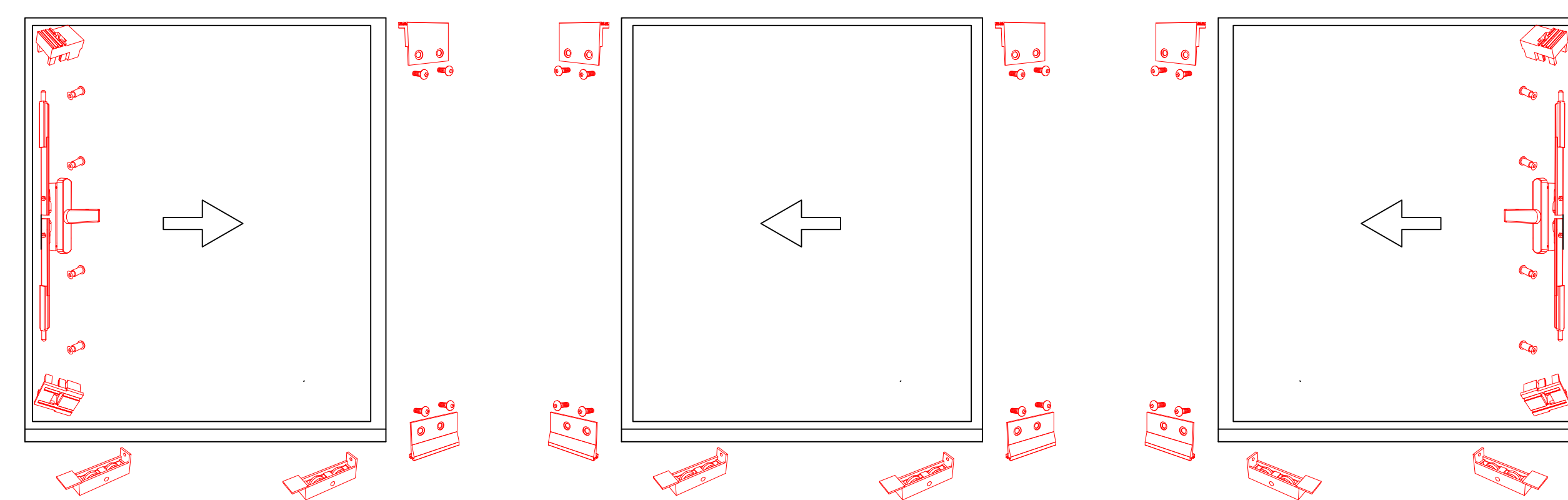
COMPONENTES DAS FOLHAS
